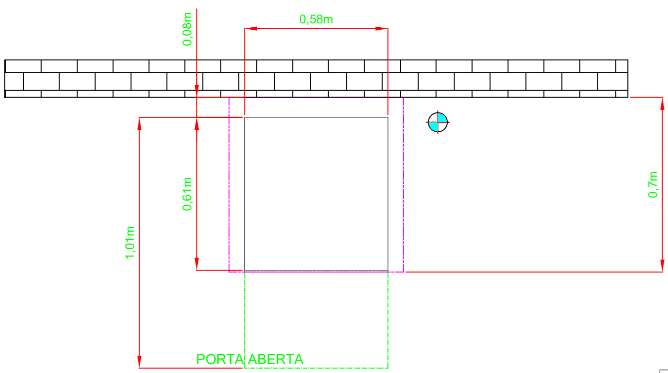
VISTA SUPERIOR
